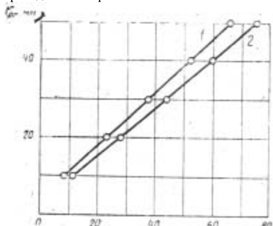
Чертеж В.1 - Градуировочные зависимости для продольных стержней диаметром 16 мм 1 - при шаге стержней s = 50 мм; 2 - при шаге стержней s = 100 мм.
